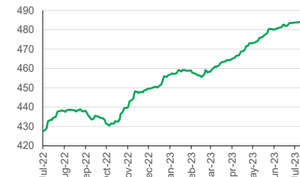
BINDO (YoY)
