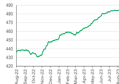
BINDO (YoY)
